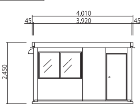
単棟 立面図
