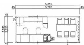
単棟 平面図
