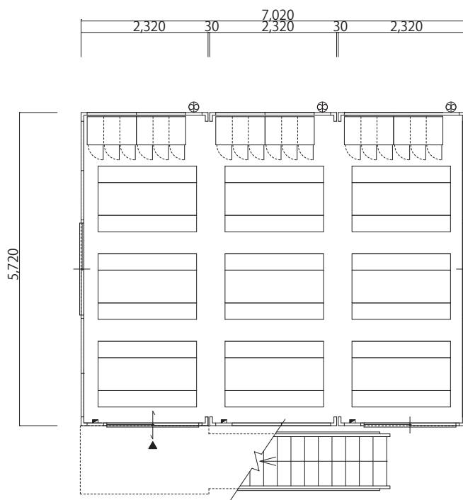
U57H(2階建3連棟)参考レイアウト
