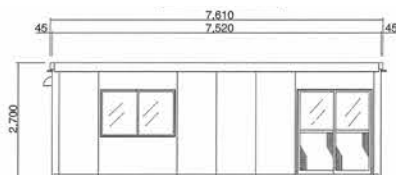
単棟 立面図
