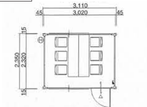
単棟 平面図
