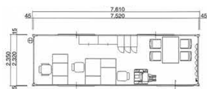
単棟 平面図
