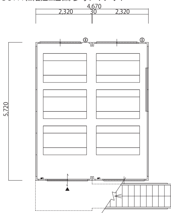
U57H(2階建2連棟)参考レイアウト
