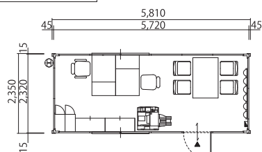
単棟 平面図
