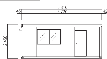
単棟 立面図
