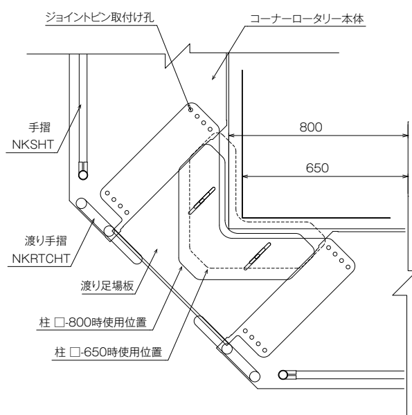
コーナーロータリー渡り足場設置例 (650~800用)
