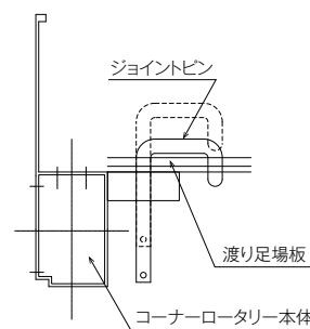
渡り足場板取付け部納まり詳細
