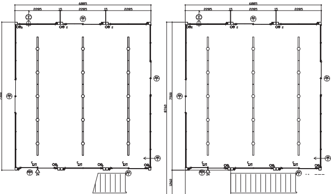
3連棟の平面図
