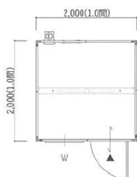
1.0間×1.0間
