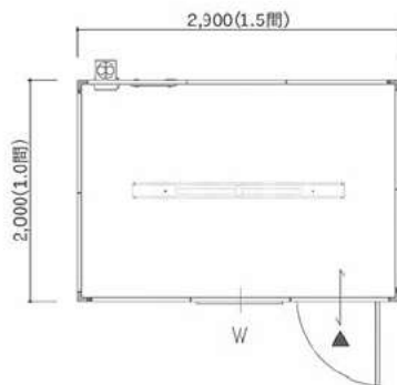
1.5間×1.0間
