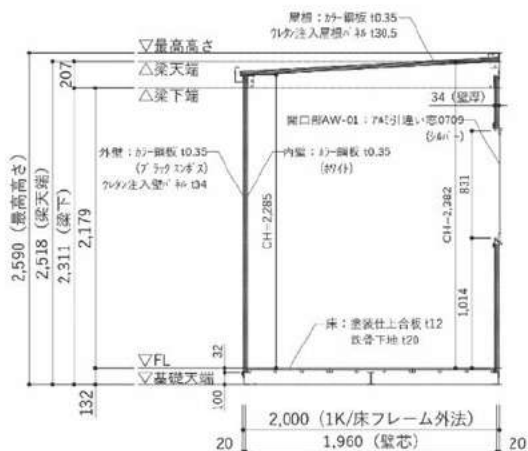
1.0間モジュール
