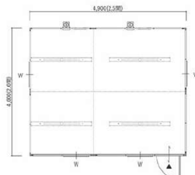
2.5間×2.0間
