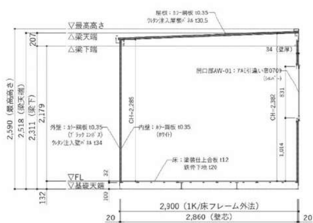
1.5間モジュール
