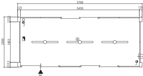
単棟 平面図
