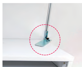
63 付けててよかった 耐震ブラケット 品番: QO-TYT2707 寸法: W70×D268×H84.5mm
