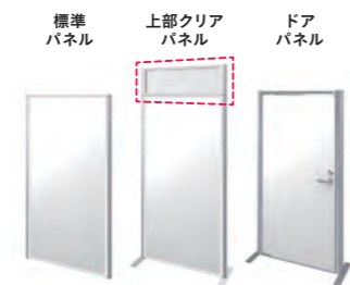
46 パーティション 品番: 標準パネル PT-SKL0918 寸法: W900×H1,800mm 品番: 上部クリアパネル PT-SKL0903C 寸法: W900×H300mm 品番: ドアパネル PT-SKLD0918 寸法: W900×H1,800mm
